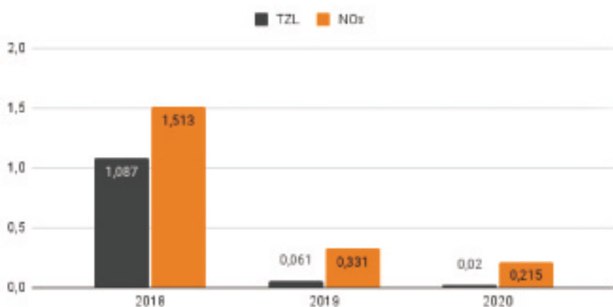
Snižování emisí tuhých znečišťujících látek do ovzduší t/rok
