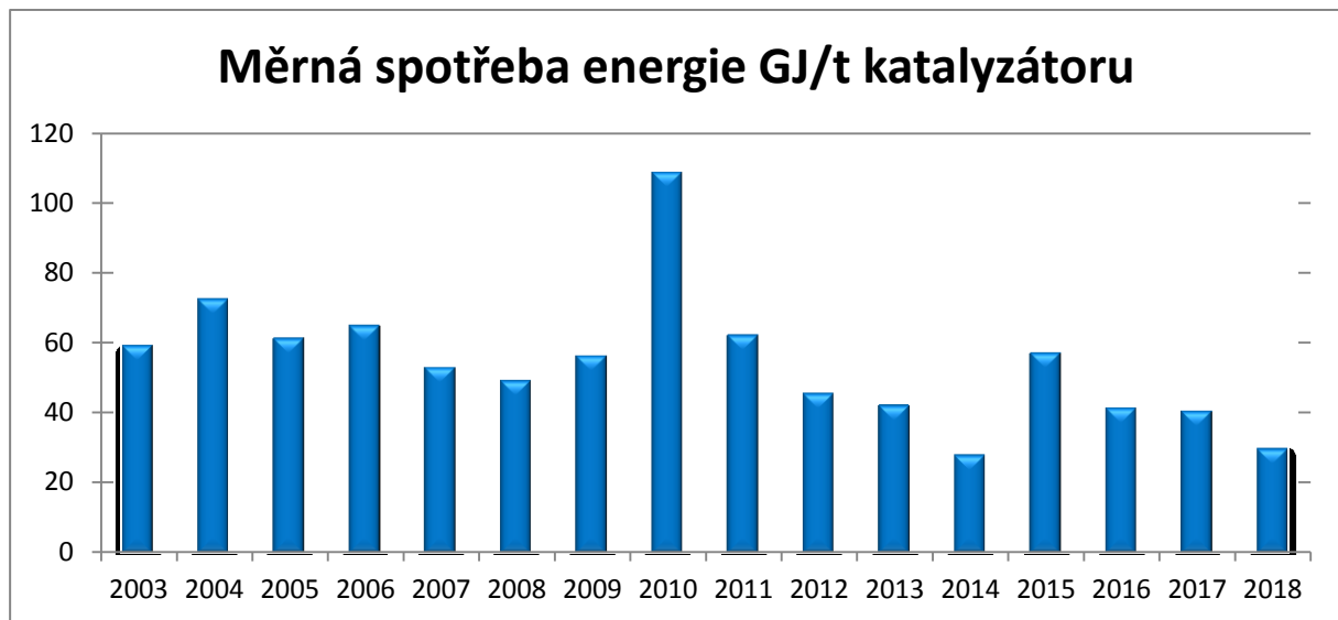
Graf 3: Měrná spotřeba energie v GJ/t katalyzátoru
