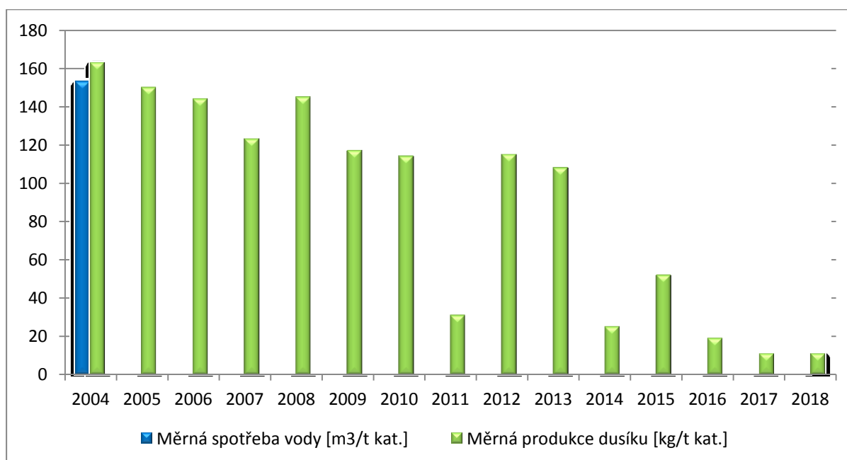
Graf 2: Vývoj měrné spotřeby vody a produkce dusíku
