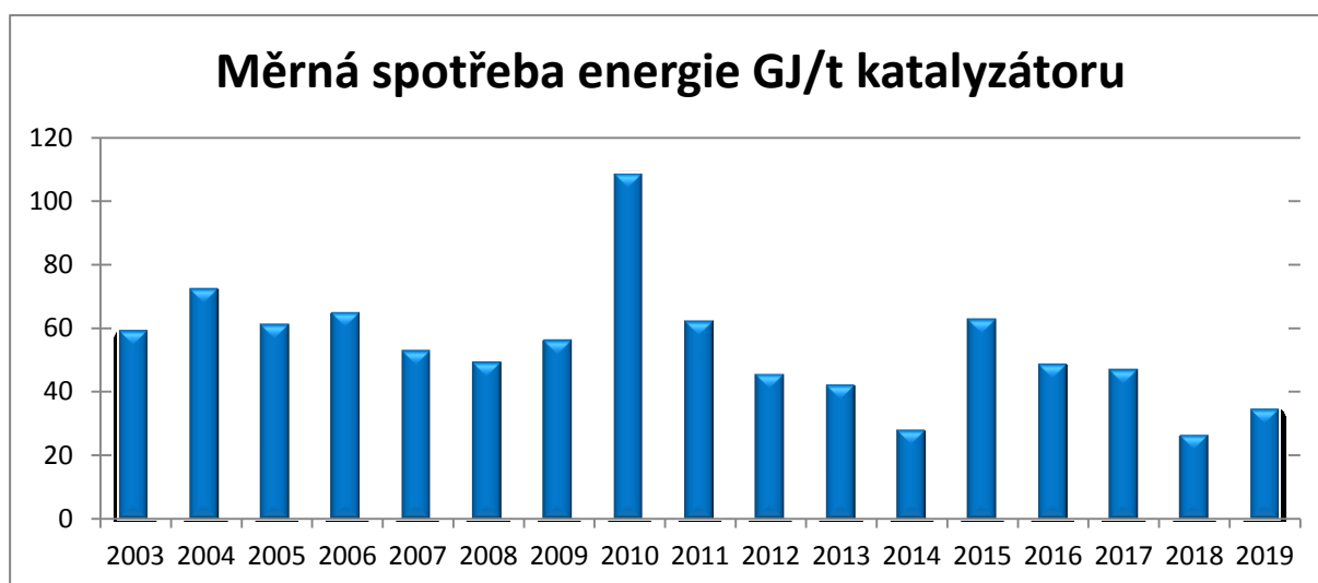
Graf 3: Měrná spotřeba energie v GJ/t katalyzátoru
